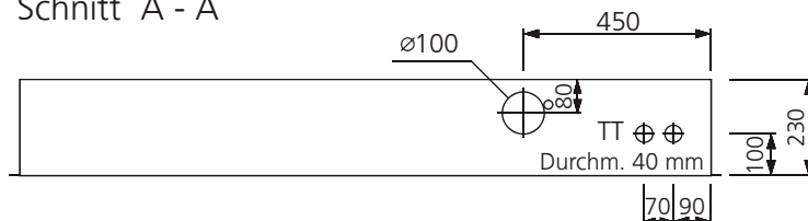
Schnitt A - A
