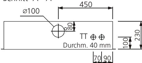
Schnitt A - A
