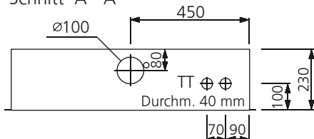
Schnitt A - A
