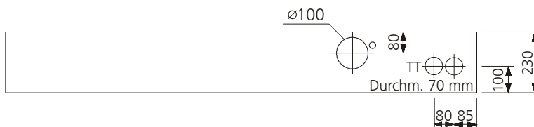
Schnitt A - A
