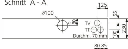
Schnitt A - A
