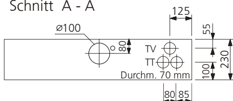
Schnitt A - A
